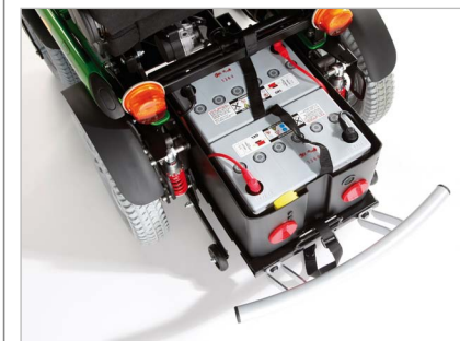
Batteriskuffe
