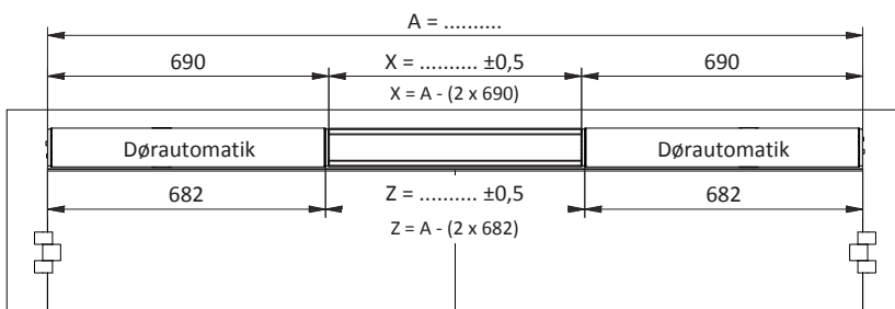
uden monteringsplade
