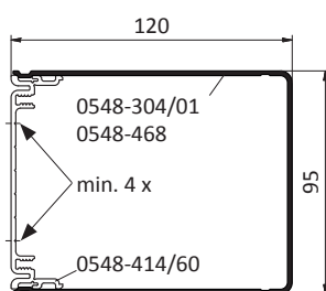
uden monteringsplade
