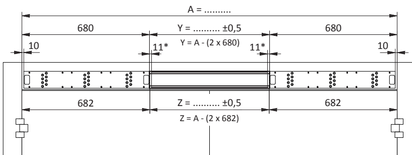
med monteringsplade
