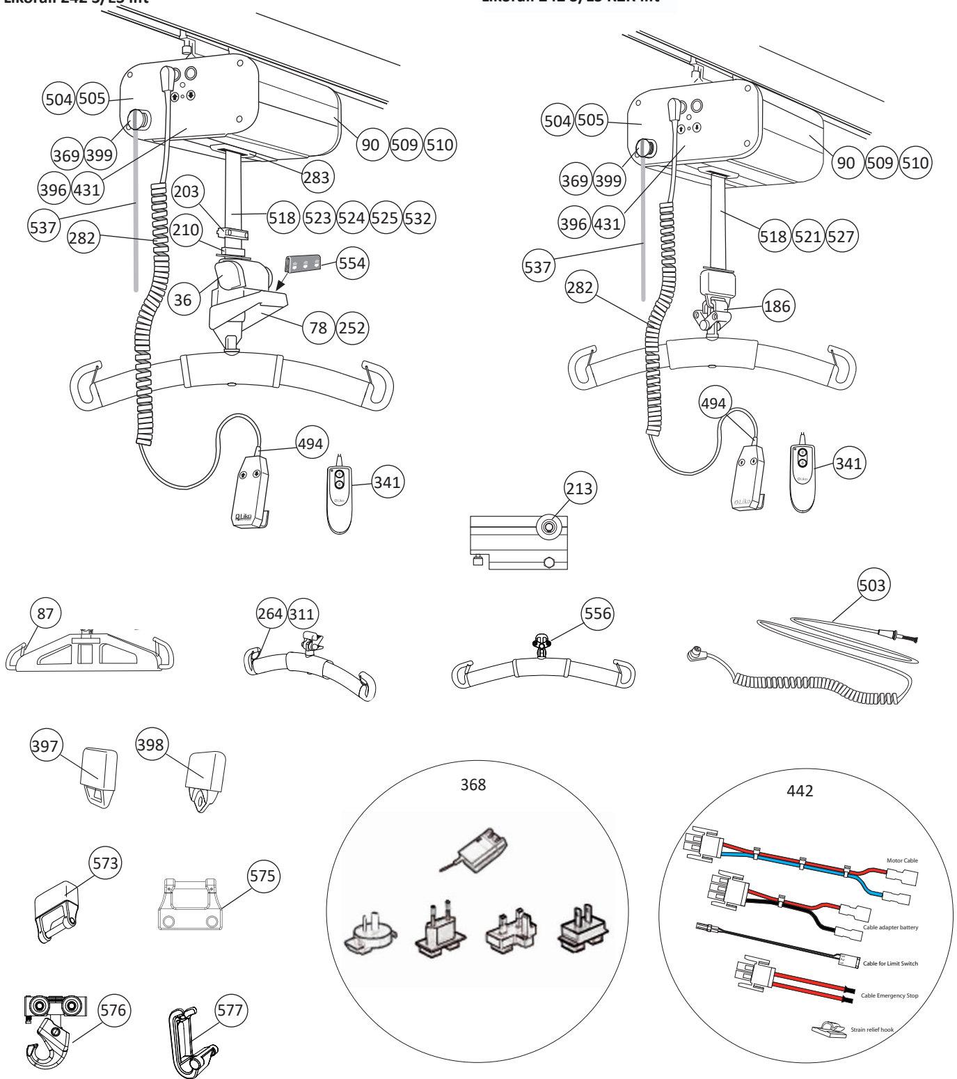
Likorall 242 S/ES lift
