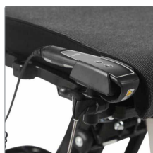
Beslag til håndbetjening Monteres foran på sædet. Håndbetjeningen klikkes let på plads vha. en magnet.
